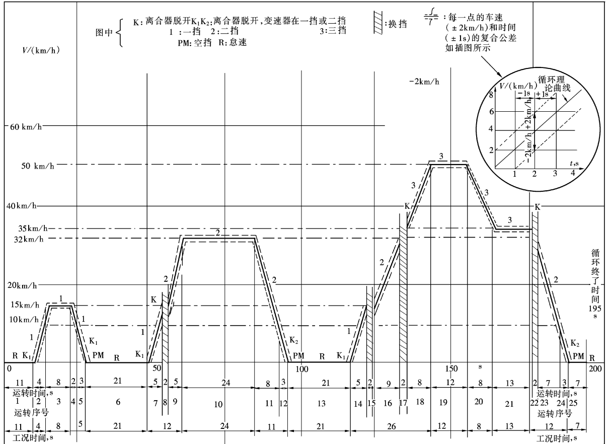
图 C.1 瞬态工况运转循环图
